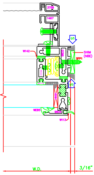
407 JAMB WW410
