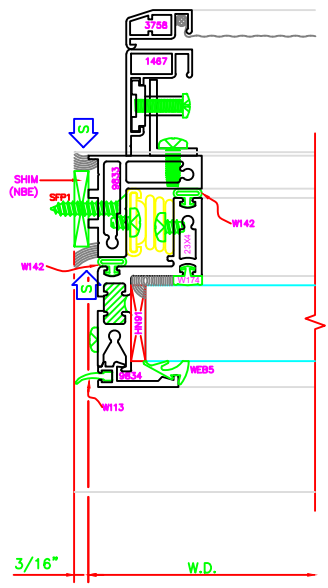
406 JAMB WW410
